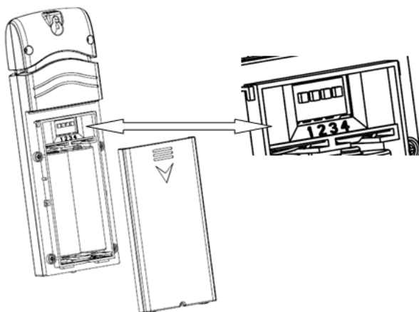
Abbildung 14 Batterieinstallation für Mehrkanalsensor
