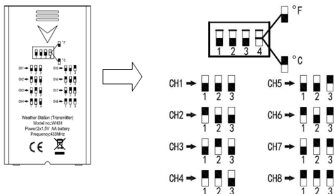
Abbildung 15: DIP-Schalter-Diagramm
