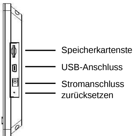
Abbildung 2: Seitenansichten der Konsole anzeigen
