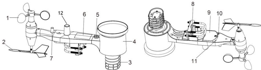
Abbildung 5: Bestandteile der Sensorbaugruppe
