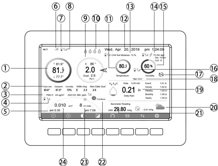
Abbildung 18: Bildschirmaufbau der Konsolenanzeige
