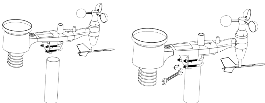
Abbildung 11: Montagediagramm des Sensorbausteins
