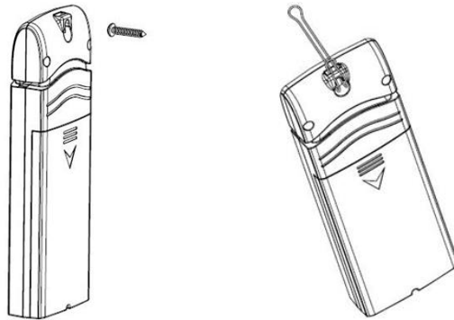
Abbildung 17: Innensensormontage
