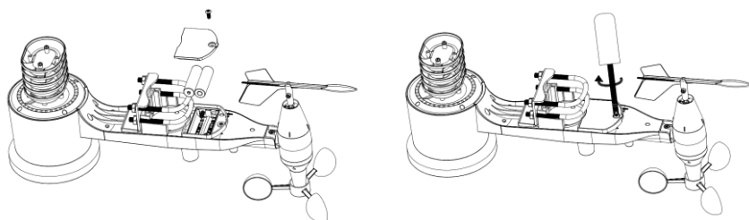
Abbildung 10: Batterieinstallationsdiagramm
