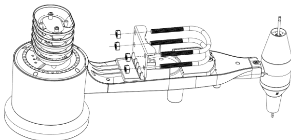
Abbildung 6: Installation des U-Bolzen
