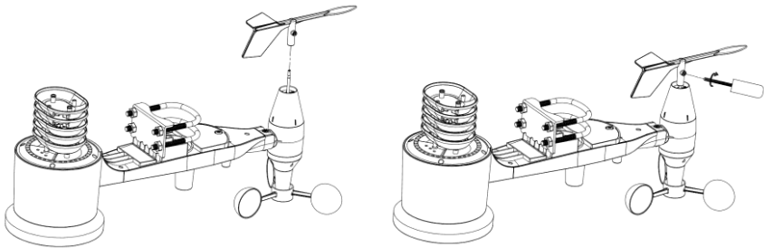
Abbildung 8: Montageplan der Windfahne
